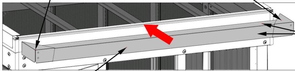
2958 (x1) EDGE TRIM
