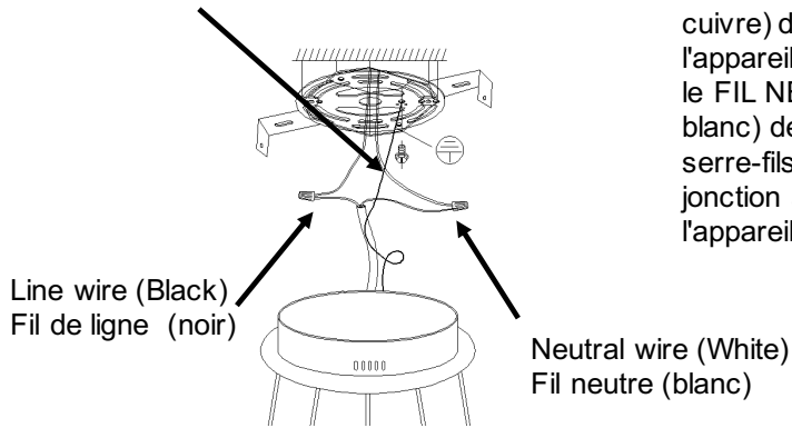
Ground wire (Copper or Green) Fil de mise à la terre (cuivre ou vert)
