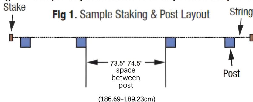
Fig. 1 : Exemple de jalonnement et de disposition des poteaux
