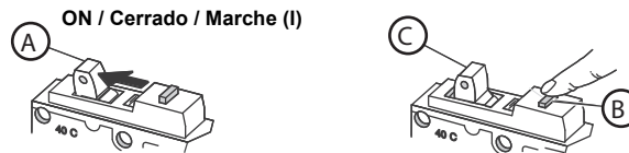
FIG. 2 : Circuit Breaker Testing / Prueba del interruptor automático / Essais du disjoncteur
