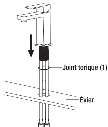
Installation éviers à 1 trou
