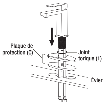
Installation éviers à 3 trous
