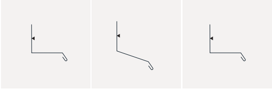
Solin de paroi latérale Finition Solin de cheminée #1
