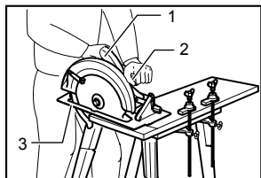
1. Poignée arrière 2. Poignée avant 3. Base
