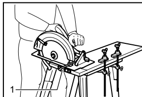
1. Garde parallèle (règle de guidage)
