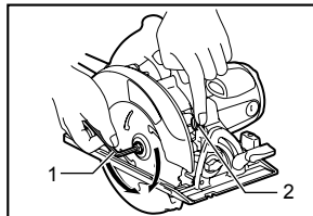
1. Clé hexagonale 2. Verrouillage de l'arbre
