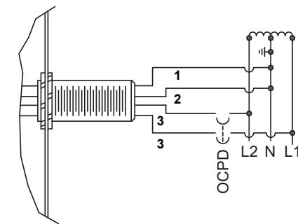
Service Entrance without Grounding Bar 120/240 V 1Ø, 3-Wire Circuit Entrada de acometida sin barra de conexión a tierra Circuito de 3 hilos, 120/240 V, 1 fase/ Barre de m.à.l.t. de l'appareil / Entrée de service sans barre de m.à.l.t. Circuit de 120/240 V, monophasé, à 3 fils
